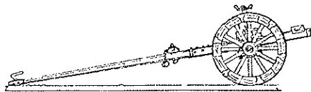
Gr. 91/ 55 Dornprotze
